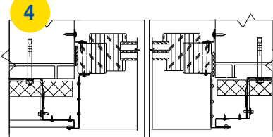
Примыкание к окну. Горизонтальный разрез.
