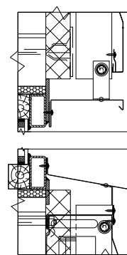
Примыкание к окну. Вертикальный разрез.
